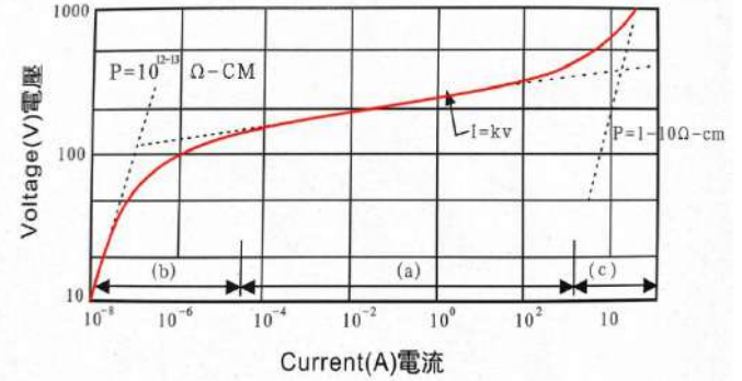
VDR
